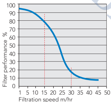
过滤性能/过滤速度
